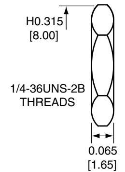
NUT
