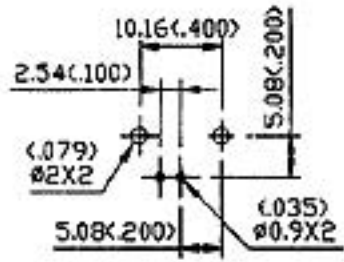
P.C.B. CONFIGURATION
